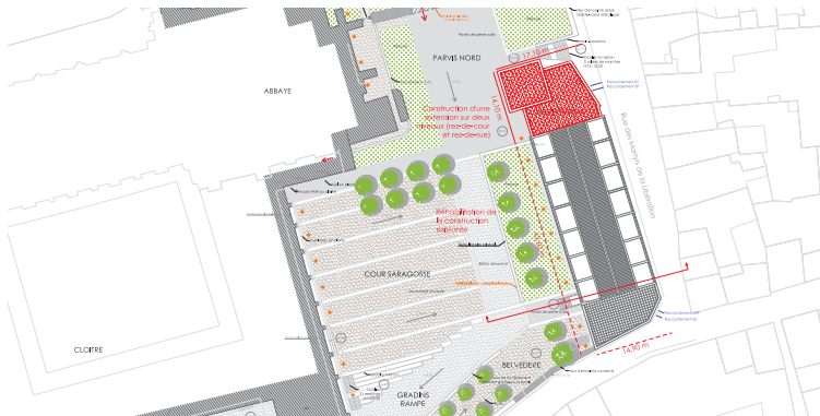
▲ Plan de masse de la médiathèque et du parvis.
